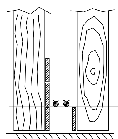
SNID A - A Í SÖKKULVEGG SÝND ERU 2 NEDSTU STEYPU-STYRKJARJÄRN Í STEYPUÓTI OFAN Á NEDSTU MÖTAVIRUM
